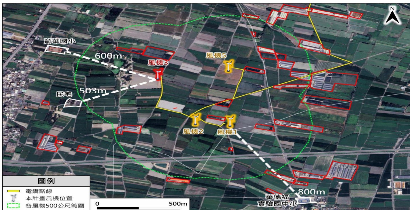
圖 1 本計畫調整後風機位置及風機淨間距示意圖
