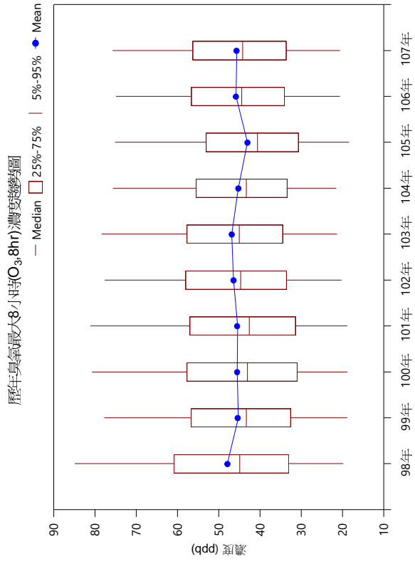
圖 3-18 (A)懸浮微粒(自動)(B)細懸浮微粒(自動)(C)細懸浮微粒(手動站)(D)細懸浮微粒(手動站-扣除陽明、三義及恆春測站) (E)二氧化硫 (F)二氧化氮 (G)一氧化氮 (H)臭氧 (I)臭氧 8 小時歷年濃度趨勢圖
