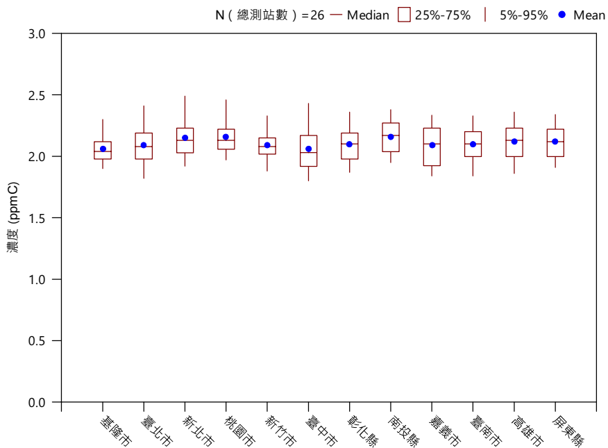
(H) 110 年行政區總碳氫化合物(THC)濃度盒鬚圖(24h)
