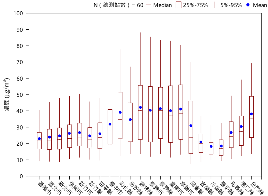
(A) 110 年行政區懸浮微粒(PM 10 )濃度盒鬚圖
