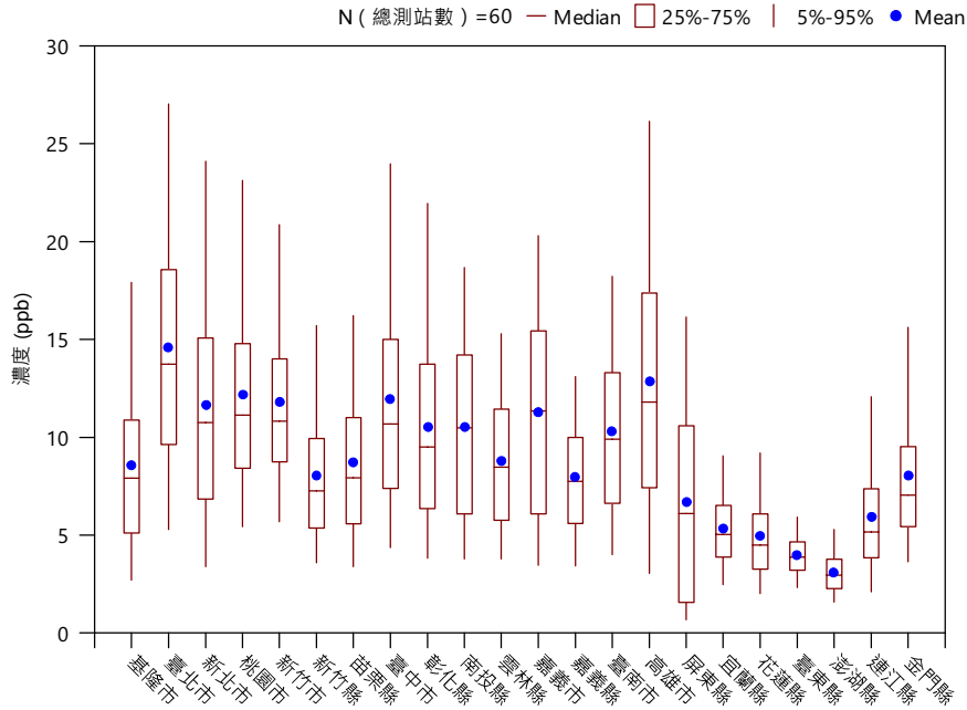
(D) 110 年行政區二氧化氮(NO 2 )濃度盒鬚圖
