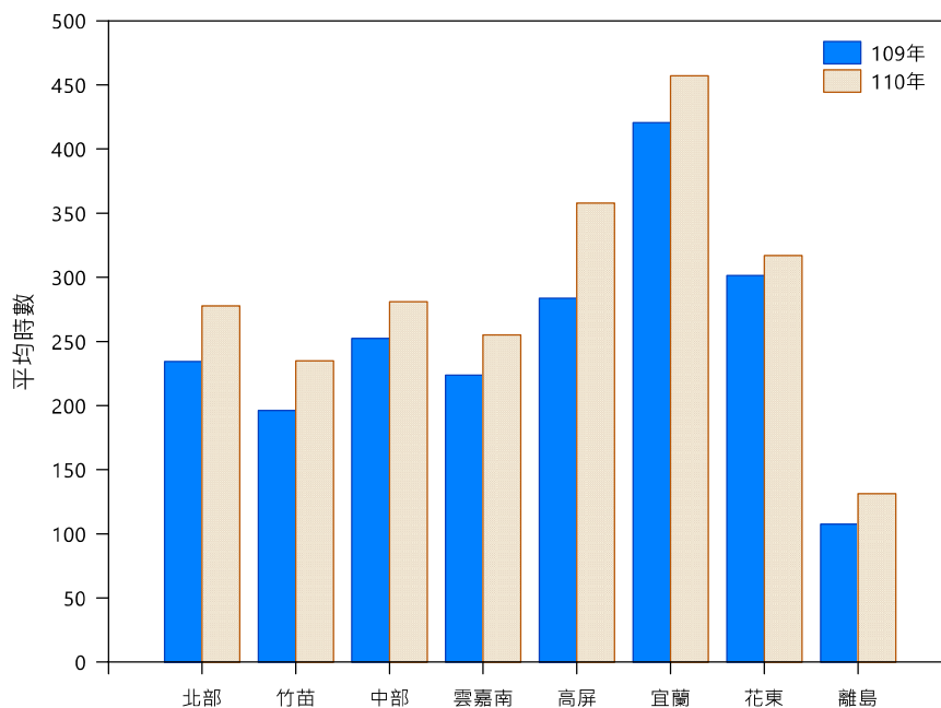
圖 3-17 109 年至 110 年各空品區及離島月風速小於 1.5 m/s 平均時數變化
