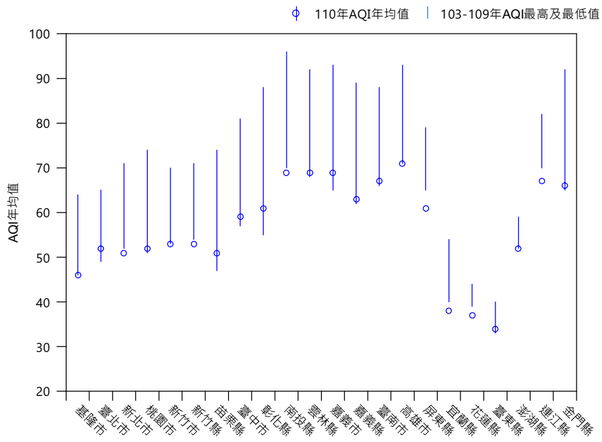
圖 3-9 行政區 110 年 AQI 年均值圖
