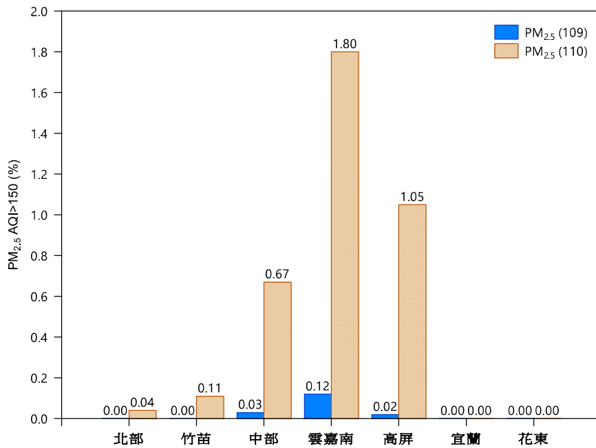
圖 3-7 109-110 年空品區 PM 2.5 AQI>150 站日數比率圖
