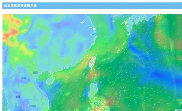
圖 2-2 空氣品質監測網三日空品區預報圖示
