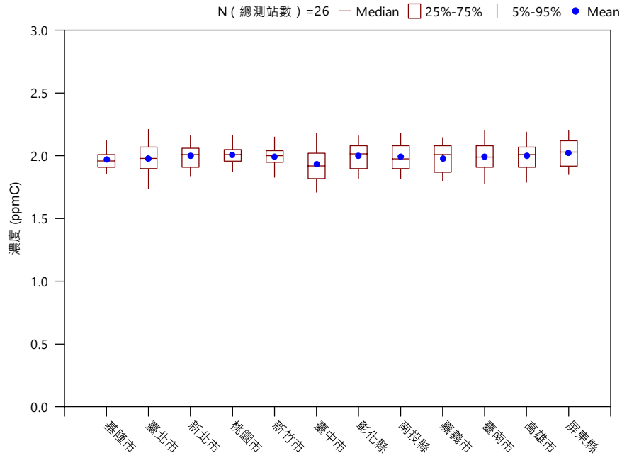
(I) 110 年行政區甲烷(CH 4 )濃度盒鬚圖(24h)
