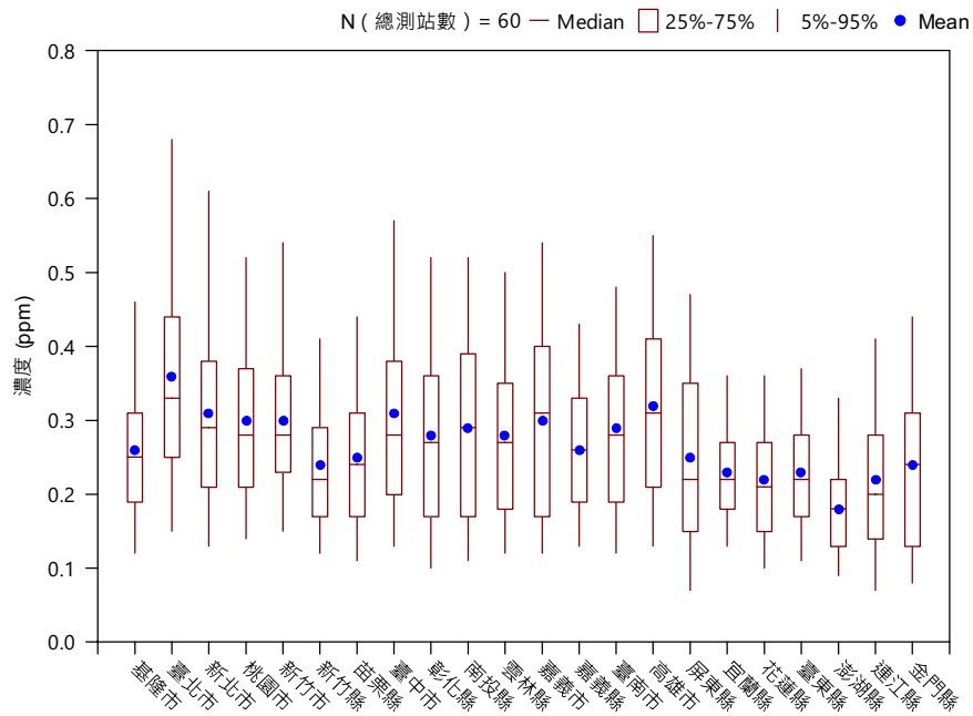
(E) 110 年行政區一氧化碳(CO)濃度盒鬚圖
