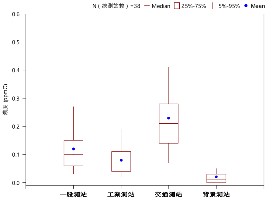
(I) 110年各測站類型甲烷(CH 4 )濃度盒鬚圖(24h)
