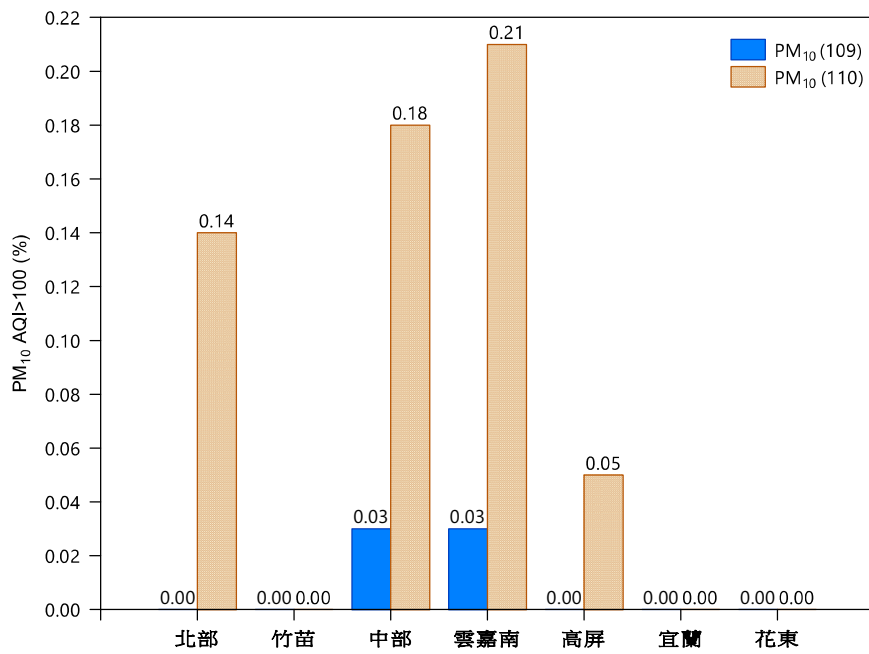
圖 3-5 109-110 年空品區 PM 10 AQI > 100 站日數比率圖
