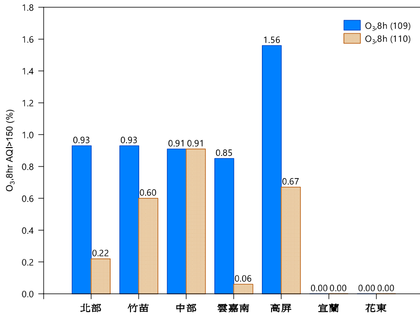
圖 3-4 109-110 年空品區 O 3,8hr AQI > 150 站日數比率圖
