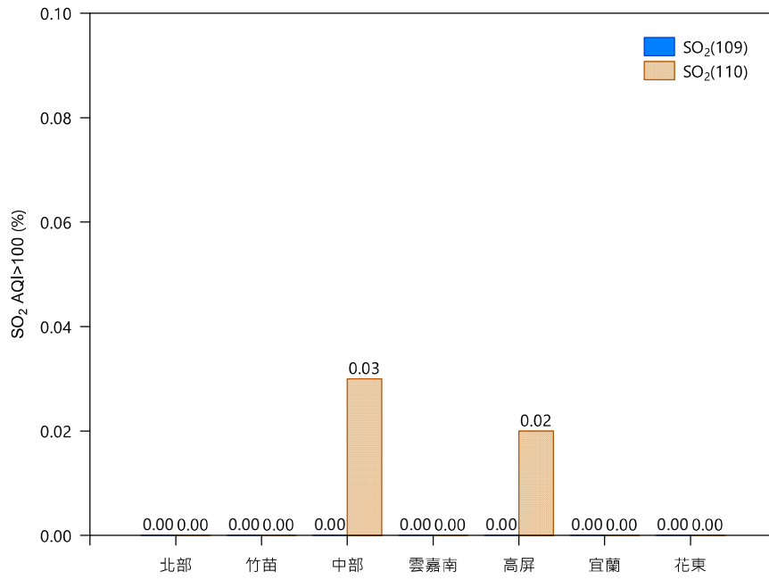
圖 3-8 109-110 年空品區 SO 2 AQI>100 站日數比率圖
