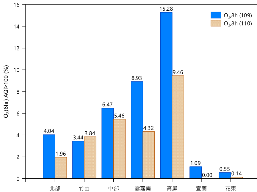
圖 3-3 109-110 年空品區 O 3,8h AQI>100 站日數比率圖
