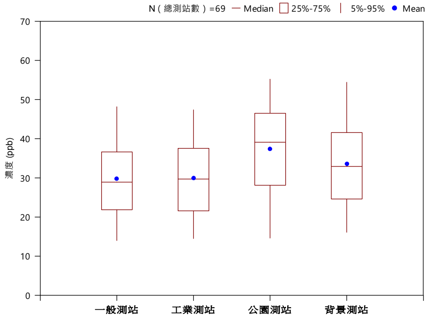
(F) 110年各測站類型臭氧(O 3 ,avg)濃度盒鬚圖
