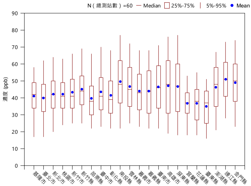
(G) 110 年行政區臭氧最大 8 小時(O 3,8h )濃度盒鬚圖
