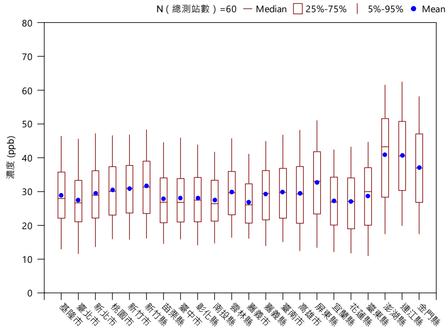
(F) 110 年行政區臭氧(O 3 ,avg)濃度盒鬚圖
