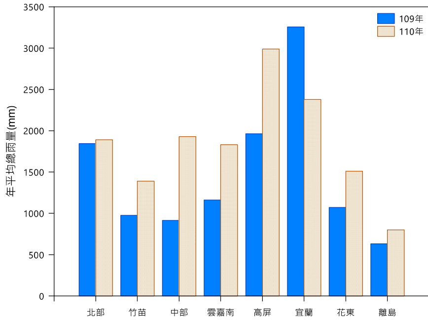
圖 3-16 109 年至 110 年各空品區及離島年平均總雨量變化
