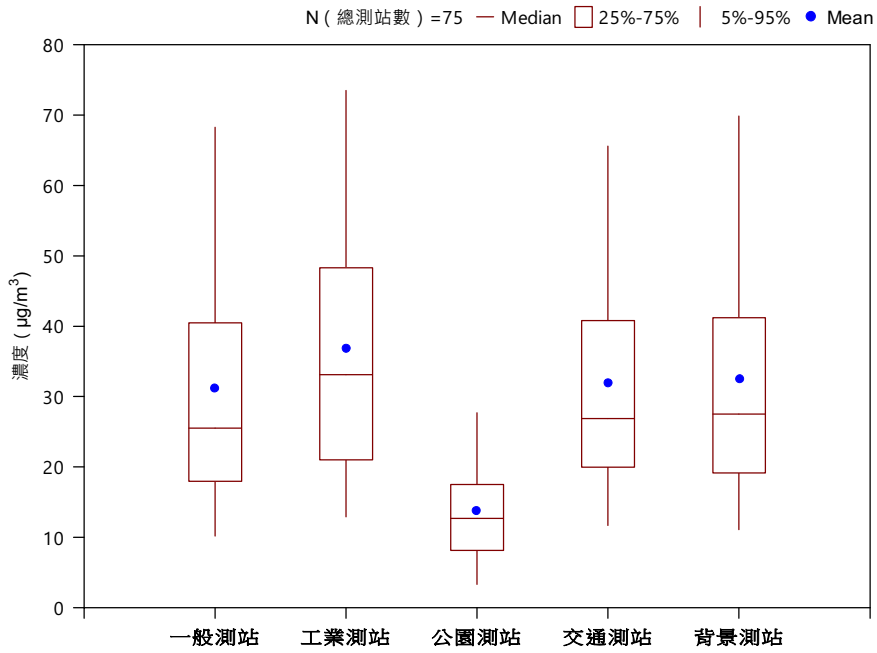
(A) 110 年各測站類型懸浮微粒(PM 10 )濃度盒鬚圖
