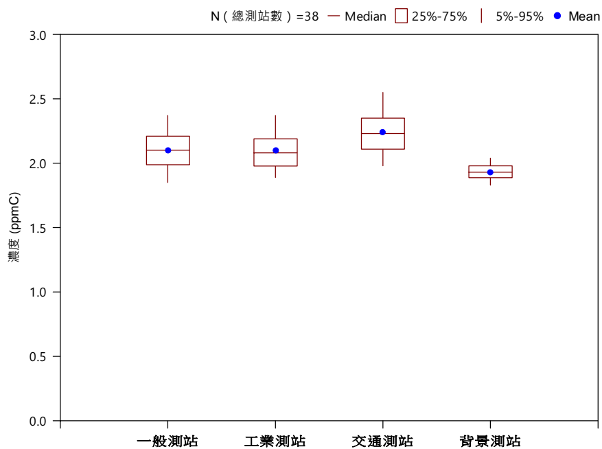
(H) 110年各測站類型總碳氫化合物(THC)濃度盒鬚圖(24h)
