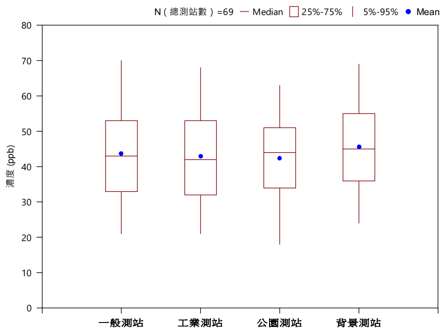
(G) 110年各測站類型臭氧最大8小時(O 3,8h )濃度盒鬚圖
