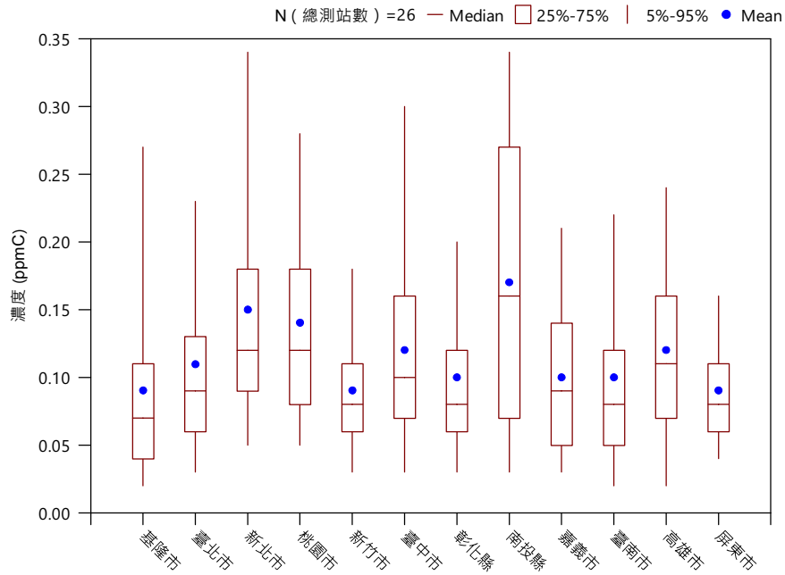
(J) 110 年行政區非甲烷碳氫化合物(NMHC)濃度盒鬚圖(24h)
