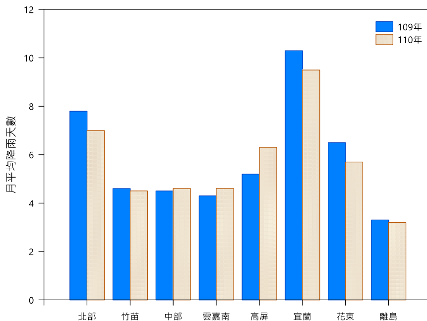
圖 3-15 109 年至 110 年各空品區及離島月平均降雨天數變化
