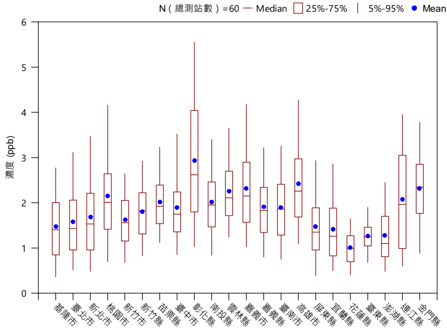
(C) 110 年行政區二氧化硫(SO 2 )濃度盒鬚圖
