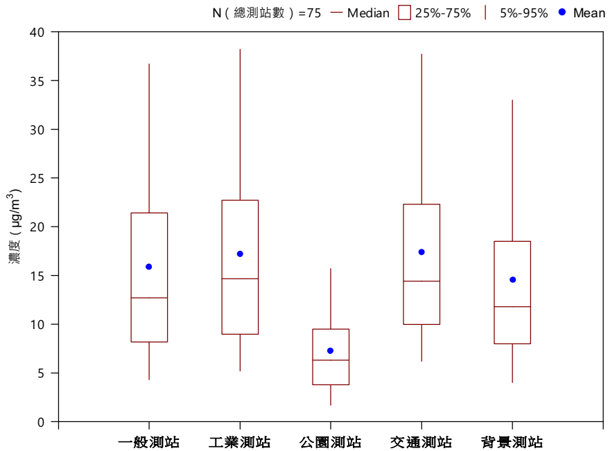
(B) 110 年各測站類型細懸浮微粒(PM 2.5 )濃度盒鬚圖
