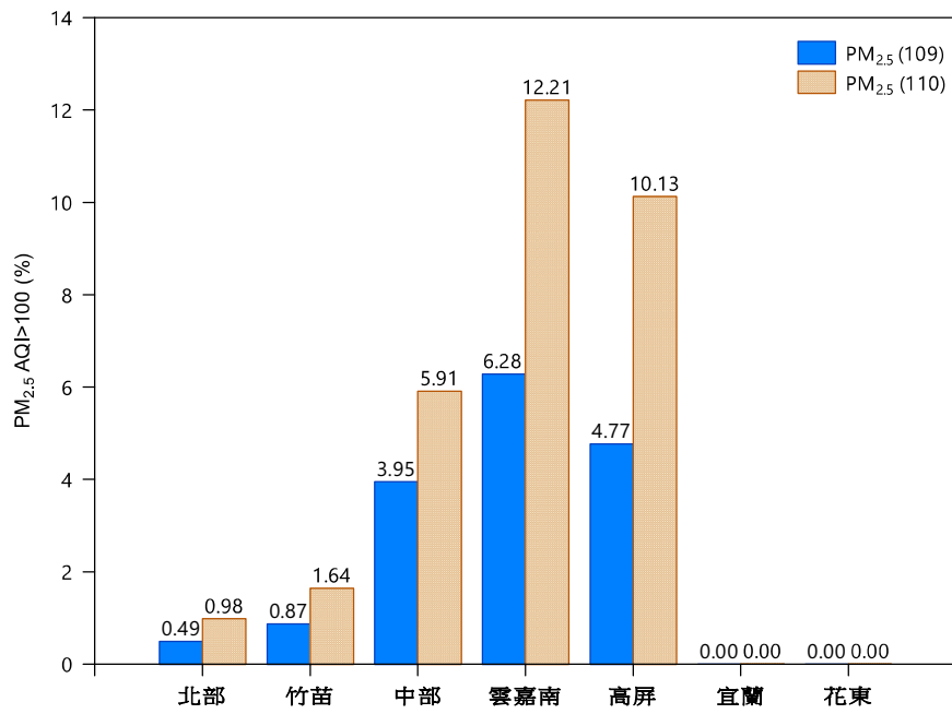
圖 3-6 109-110 年空品區 PM 2.5 AQI>100 站日數比率圖
