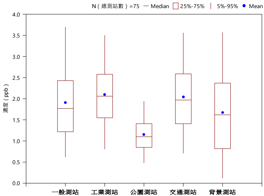
(C) 110年各測站類型二氧化硫(SO 2 )濃度盒鬚圖
