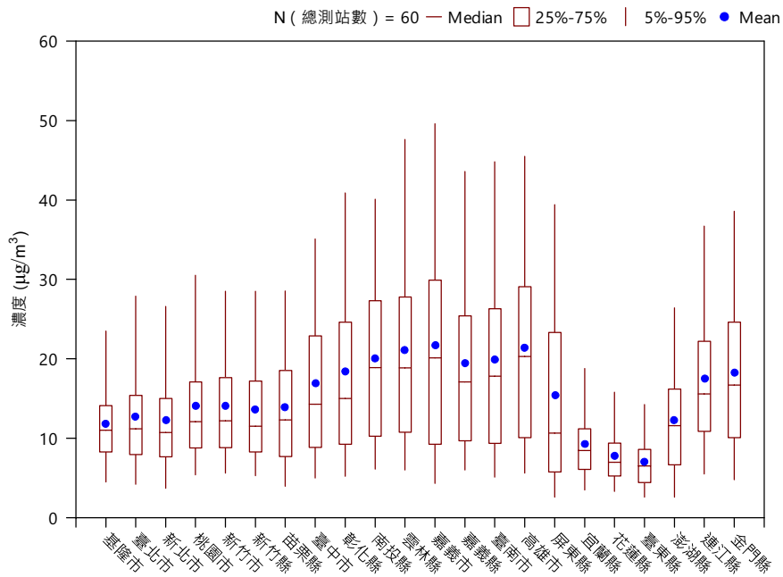
(B) 110 年行政區細懸浮微粒(PM 2.5 )濃度盒鬚圖
