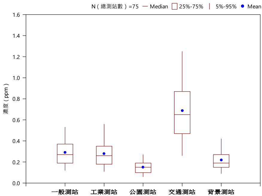
(E) 110年各測站類型一氧化碳(CO)濃度盒鬚圖
